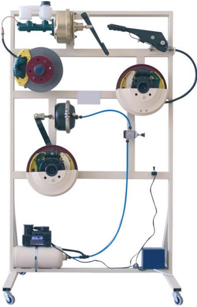
Hidrolik Fren Sistemi Seti
