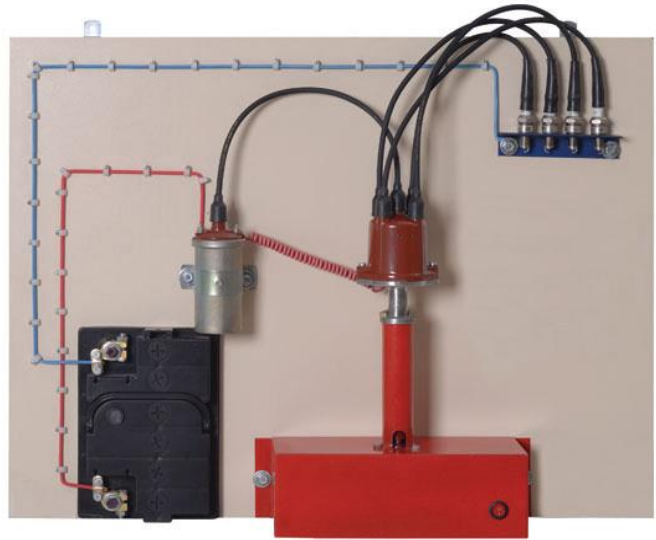
Ateşleme Sistemi Seti
